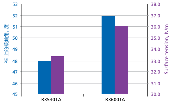
三官能多元醇 Polyol R3530 和 Polyol R3600 的丙烯酸酯在 PE 上的表面张力和接触角
