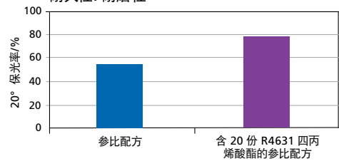
200 次 scotch-brite 擦拭后的 20° 保光率表明 Polyol R4631 的丙烯酸酯可改善耐刮擦性
